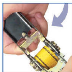
Mecanismo de rápida liberación.
